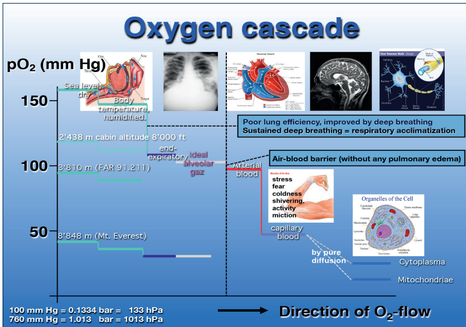
Bild 2: Oxygen cascade
